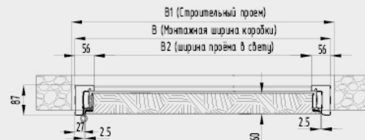
ДВЕРНАЯ КОРОБКА ДЛЯ ВРЕЗНОГО МОНТАЖА
